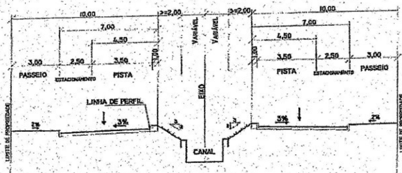
SEÇÃO-TIPO EM VIAS ARTERIAIS COM CANALIZAÇÃO
