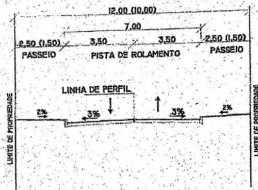
SEÇÃO-TIPO EM VIAS LOCAIS
